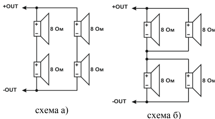
Рис. 8 Вариант 2 подключения PO
