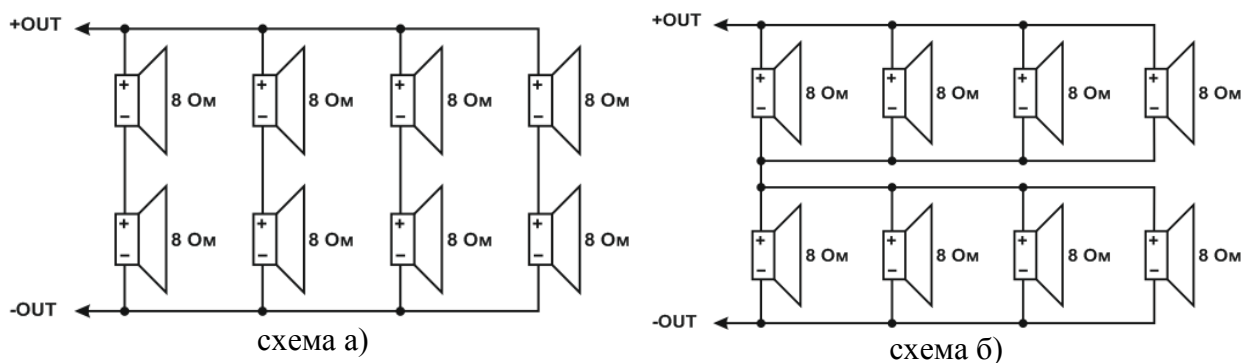
Рис. 7 Вариант 1, подключения PO.
