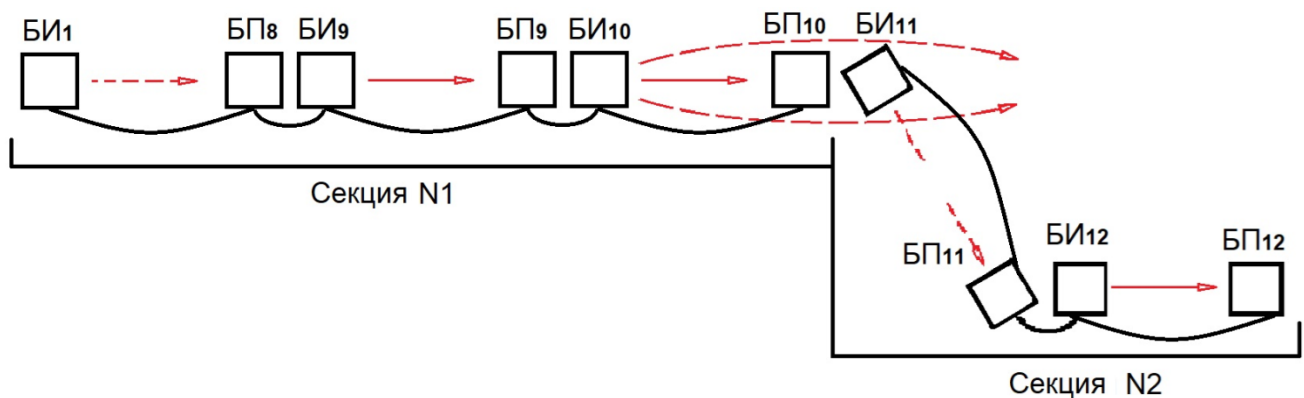
а) Вариант 2 - правильно установленные извещатели
