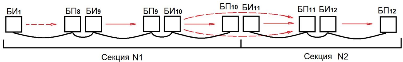
а) Вариант 1 - неправильно установленные извещатели
