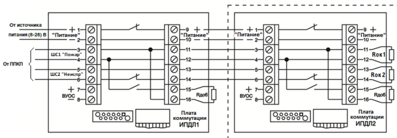
а) Схема подключения извещателя к ППКП
