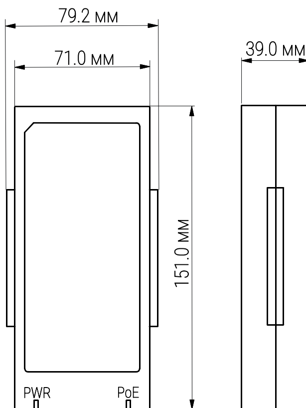
Рисунок 4.1 – Габаритные размеры
