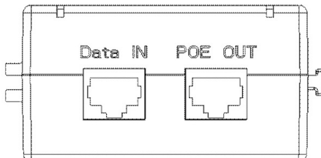
Рисунок 3.1 – Передняя панель
