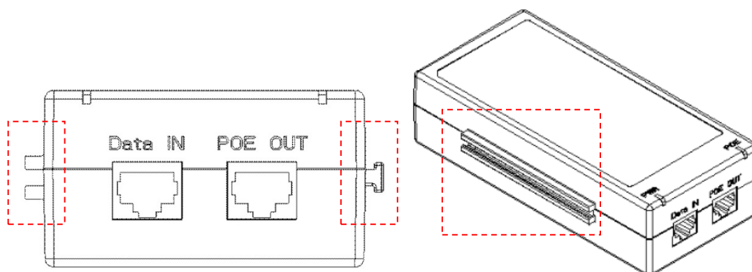
Рисунок 4.3 – Передняя панель
