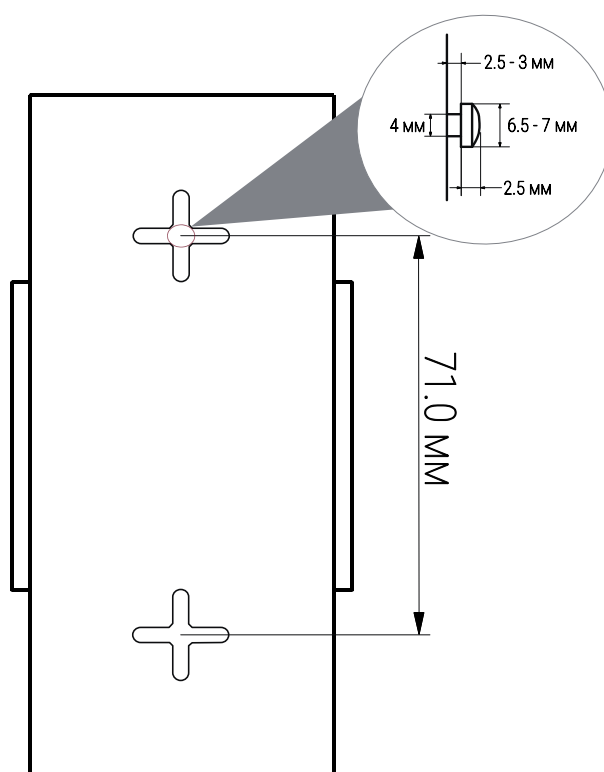
Рисунок 4.2 – Размеры и размещение
