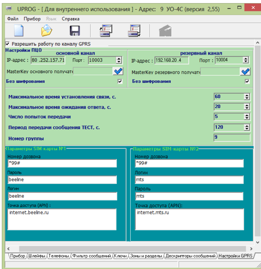
Рисунок 21. Настройка GPRS
