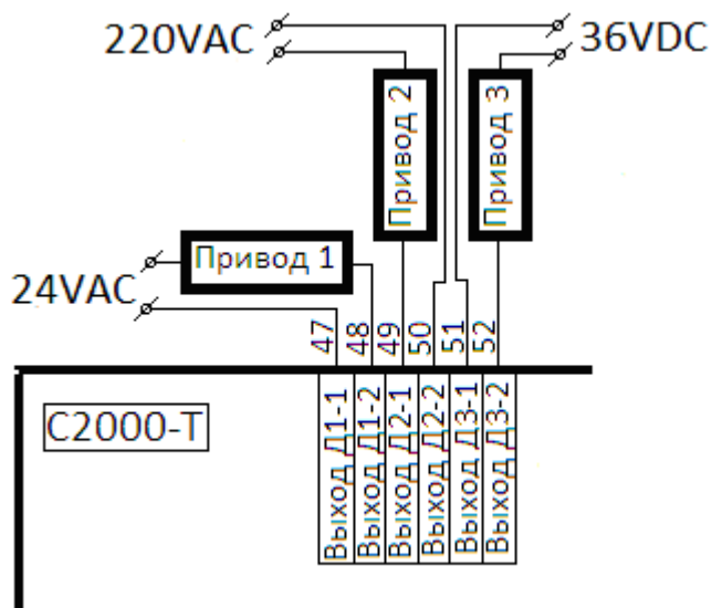
Рисунок 3.9 Подключение ИМ к дискретным выходам
