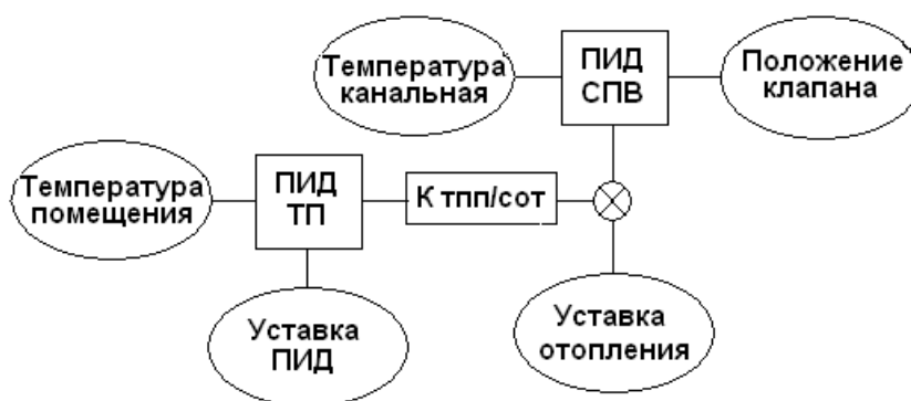
Рисунок 4.5 Каскадное регулирование в СОт
