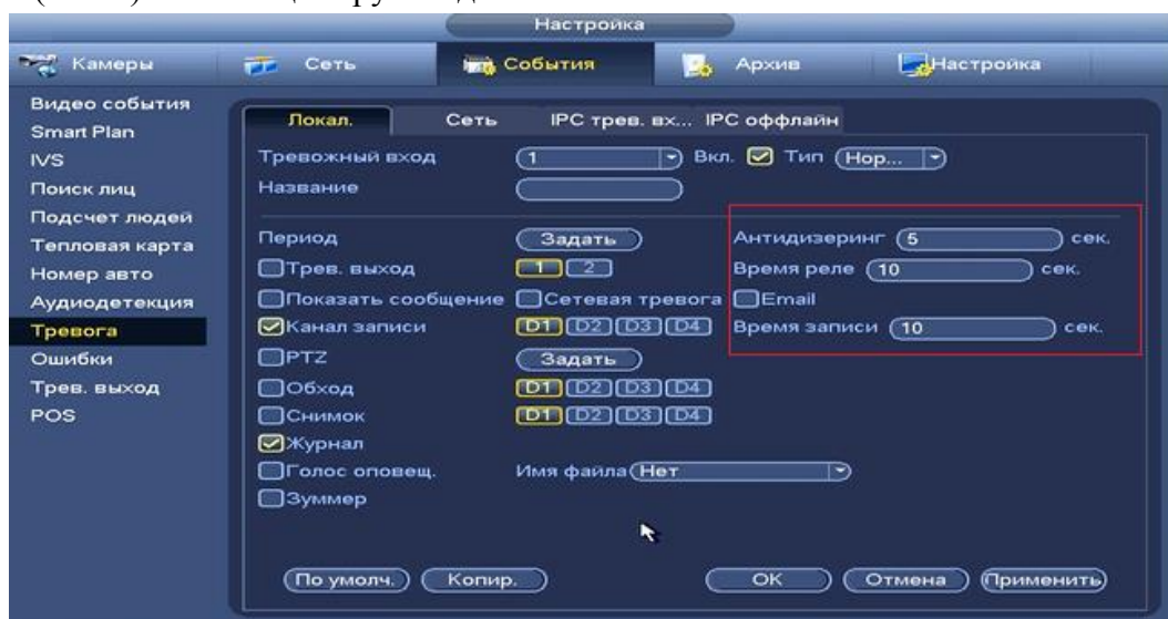
Рисунок 8.3.3.9.1.5 Установка настроек.
