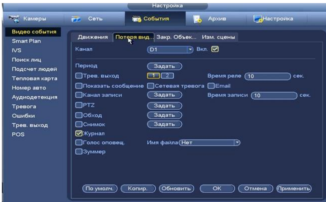
Рисунок 8.3.3.1.3.5 Установка настроек.
