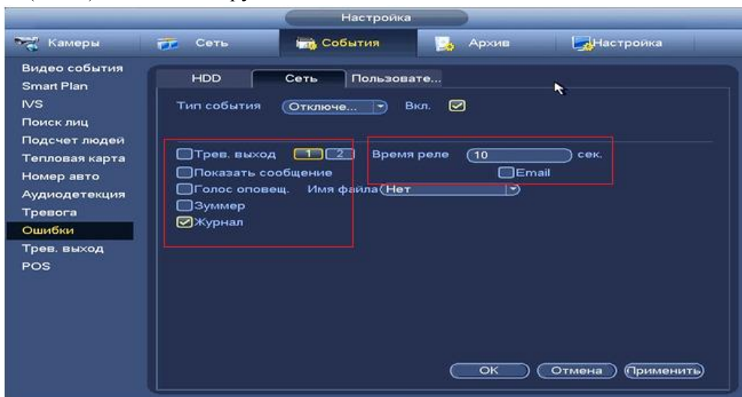
Рисунок 8.3.3.10.2.2 Установка настроек.
