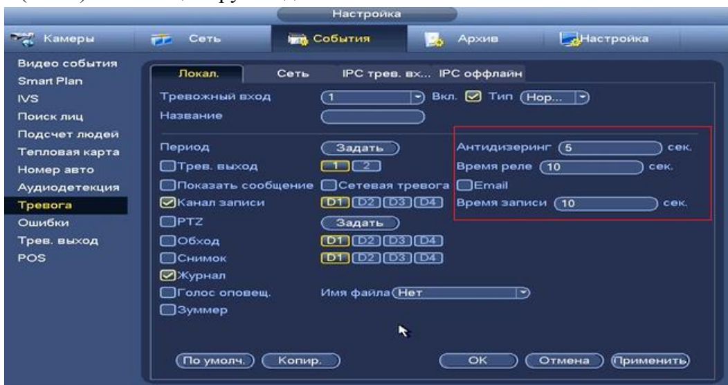
Рисунок 8.3.3.9.1.5 Установка настроек.
