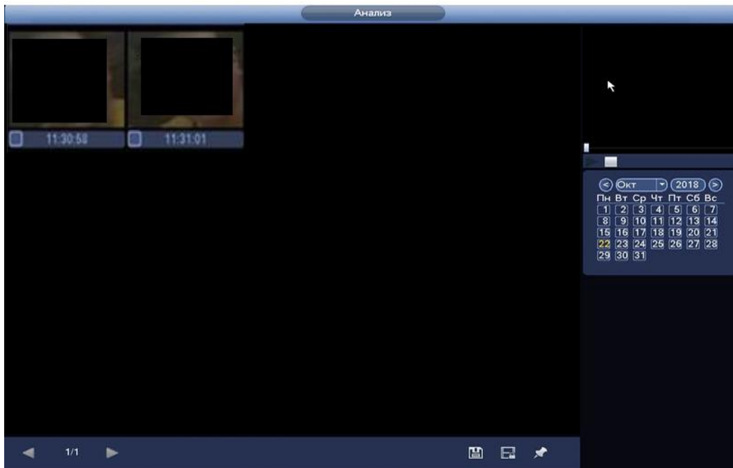
Рисунок 8.1.2.2.1 Распознавание лиц.
