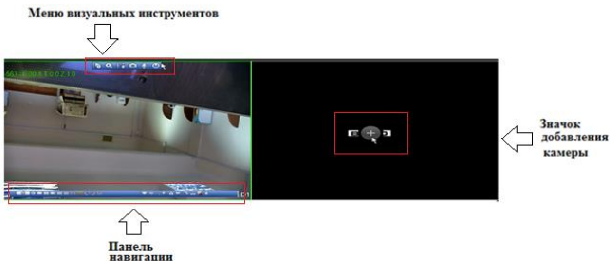
Рисунок 7.1.1.1 Добавление IP-камер.
