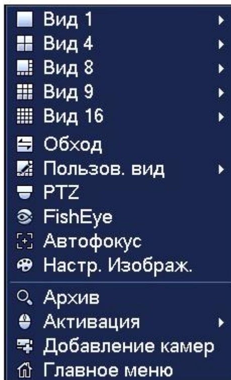
Рисунок 7.1 Контекстное меню.
