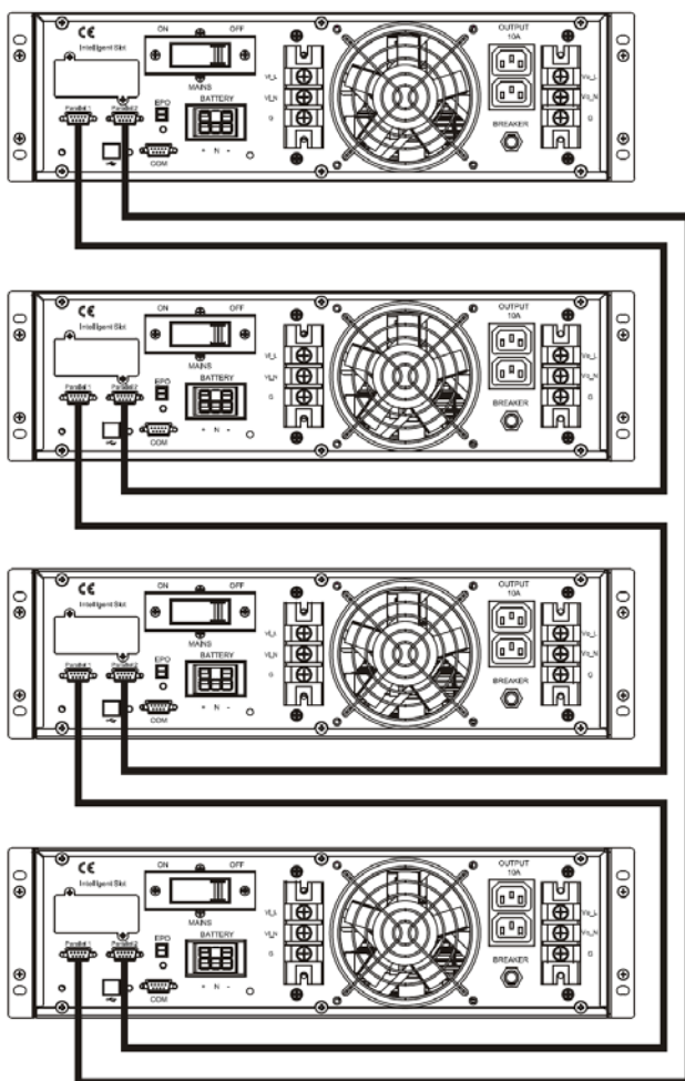
Рисунок 26 — объединение изделий в систему параллельного резервирования.
