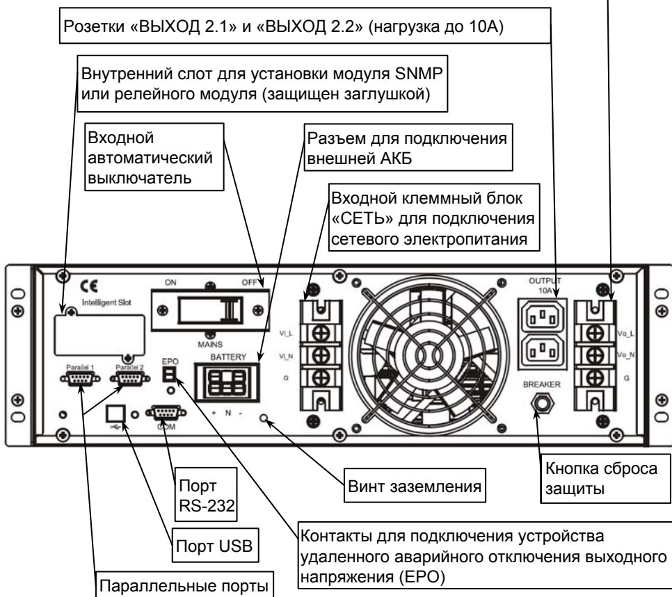
Рисунок 2 — общий вид задней панели изделия со снятыми защитными крышками
