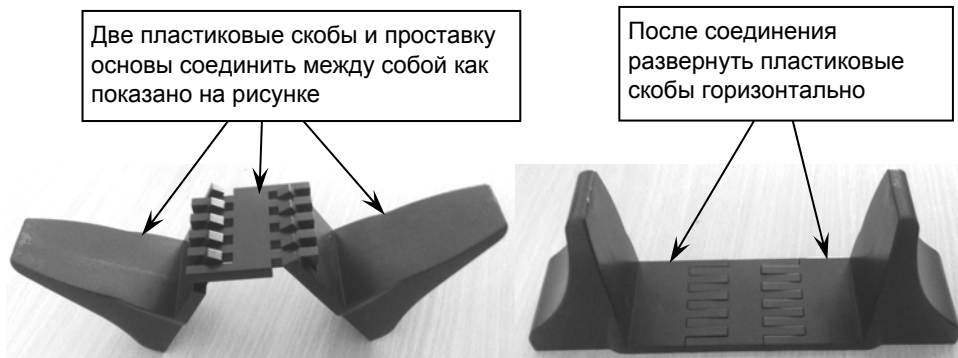
Рисунок 23 - пластиковая основа для вертикальной установки изделия
