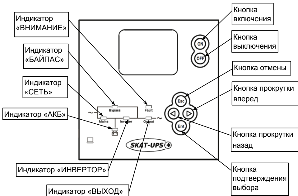
Рисунок 3 — передняя панель изделия при монтаже в горизонтальном положении
