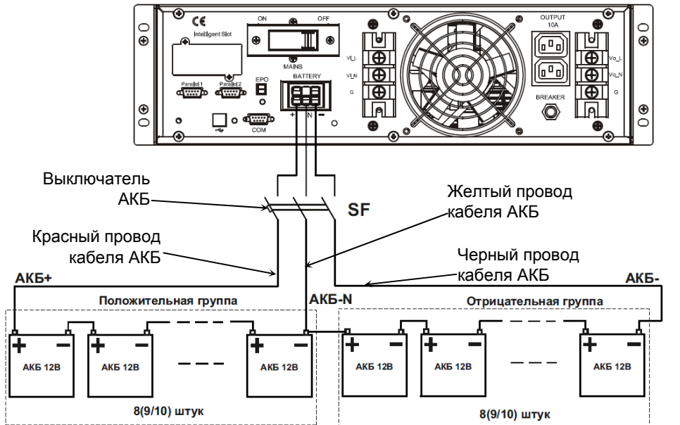
Рисунок 24 — схема монтажа аккумуляторной батареи.
