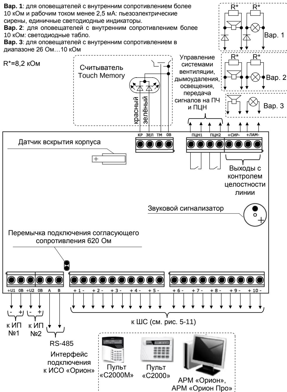
Рисунок 4. Схема внешних соединений прибора
