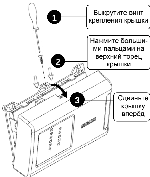
Рисунок 2. Снятие крышки прибора
