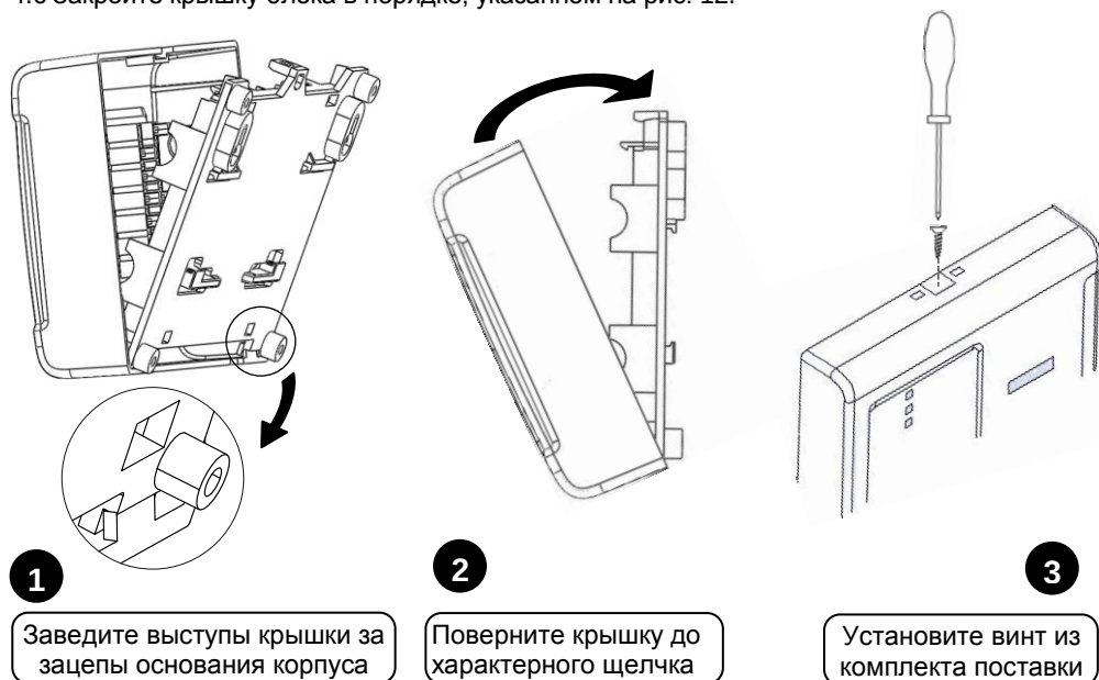
Рисунок 12. Установка крышки блока
